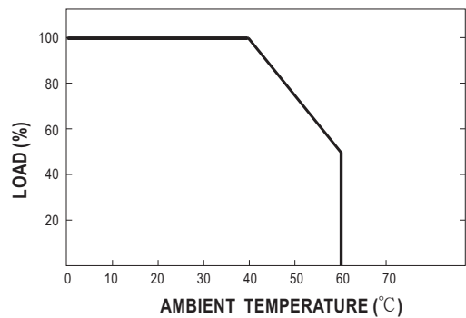
AMBIENT TEMPERATURE (°C) CURVE 1
