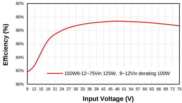
CQB150W8-36S05 Eff Vs Vin @25 Deg. C
